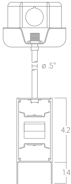
Pendant stem
