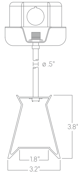
Pendant stem
