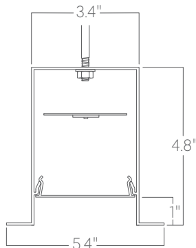
F flange
