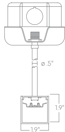
Pendant stem
