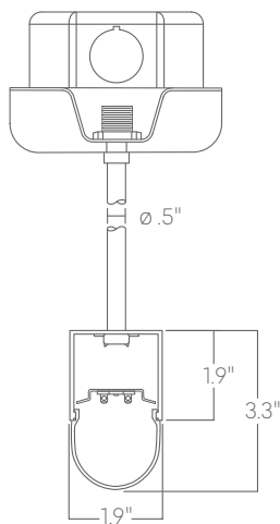
Pendant stem
