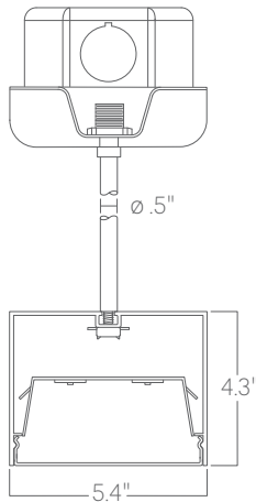
Pendant stem
