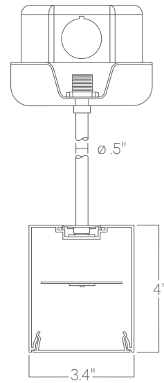
Pendant stem
