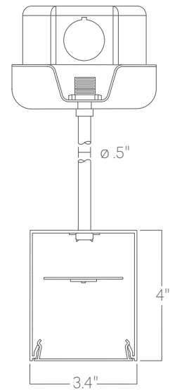
Pendant stem
