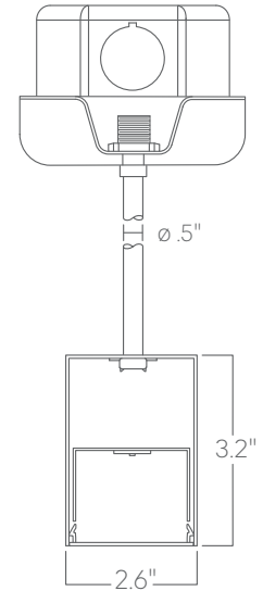
Pendant stem
